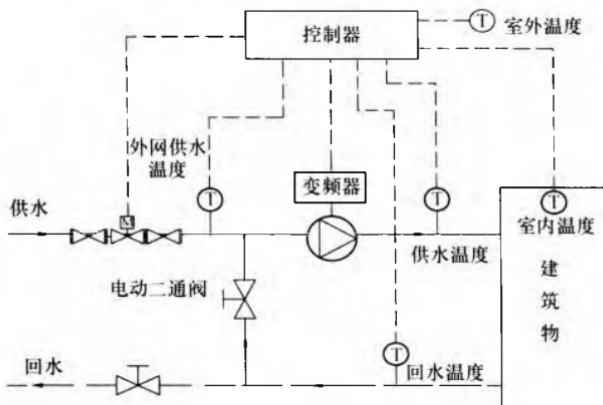
图 F.0.4 楼前混水系统示意图
