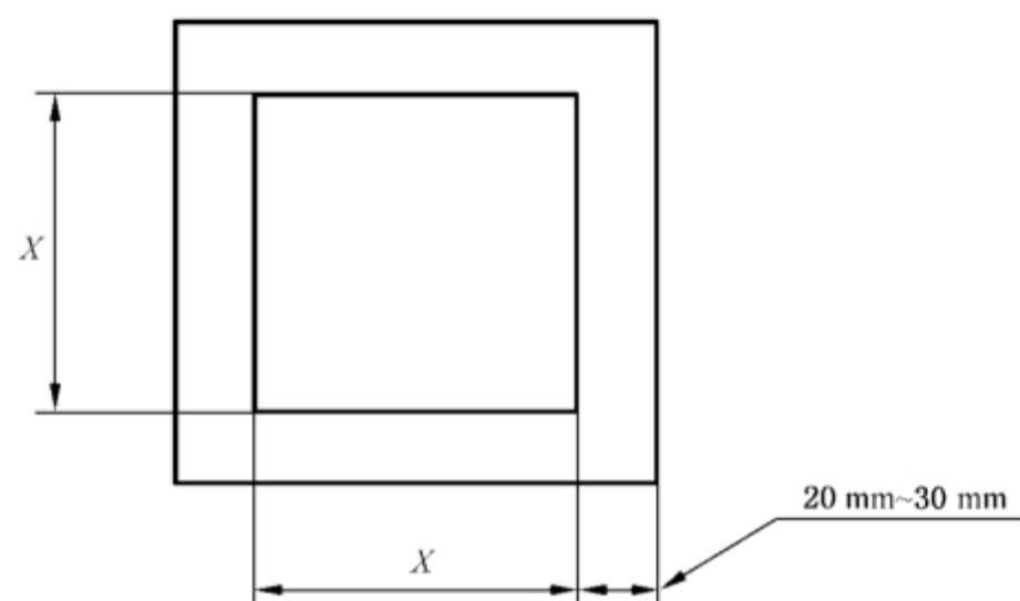
图 B.1 尘埃采样模板
